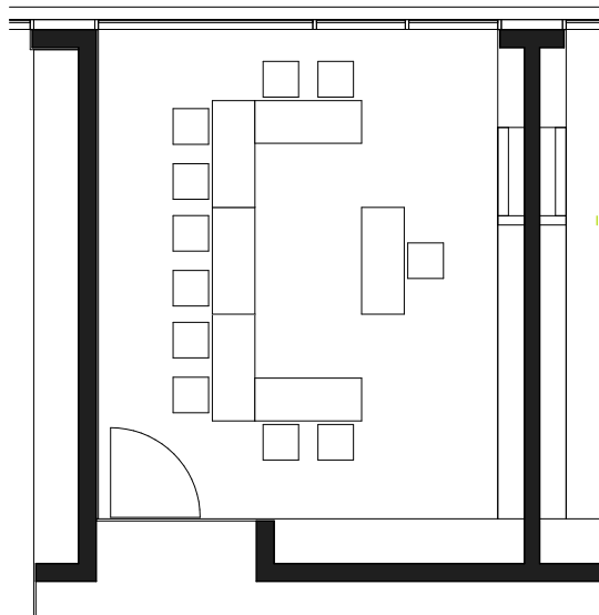
□ U 10+1 7 Tische 150/60, 13 Stühle
