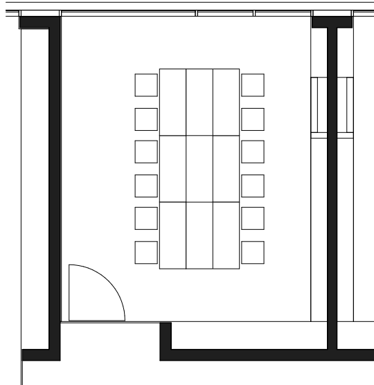
Block 12/8 8 Tische 150/60, 12 Stühle
